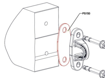
Figura 8. Colocación de la almohadilla de EP DM bajo el anclaje IRUDEK PRO 4
