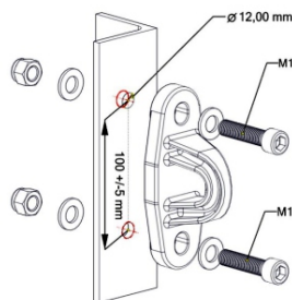
Figura 5. Montaje de conectores atornillados con el punto de anclaje a la estructura de acero
