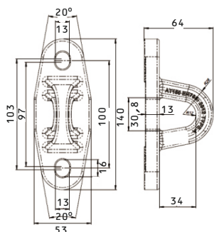
Figura 2. Dimensiones generales de IRUDEK PRO 4
