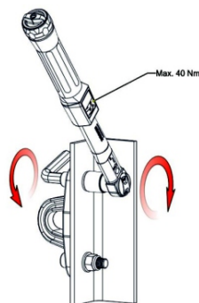
Figura 6. Forma de apriete del punto de anclaje a la estructura de acero mediante una llave dinamométrica
