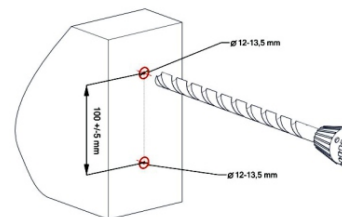
Figura 9. Taladrado de los orificios de anclaje IRUDEK PRO 4
